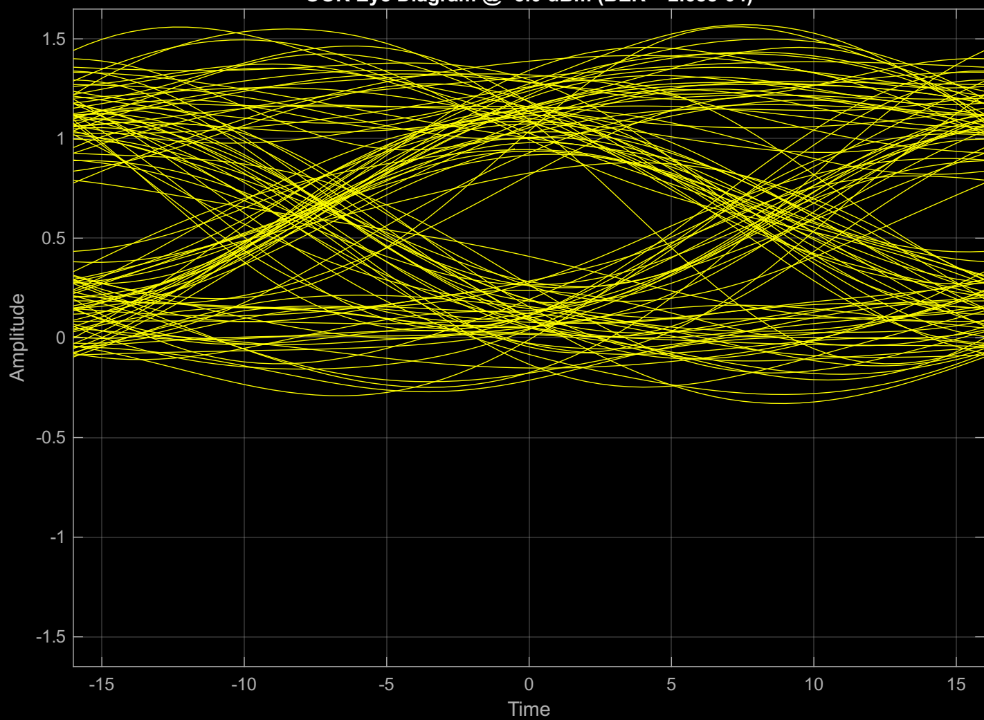
OOK Eye Diagram @ -5.0 dBm (BER \approx 2.68\text{e-}04 )
